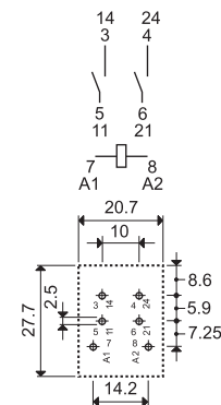
56.42-0300 Вид сбоку
