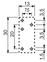
95.13.2 Вид сбоку
