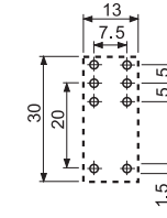
95.15.2 Вид сбоку
